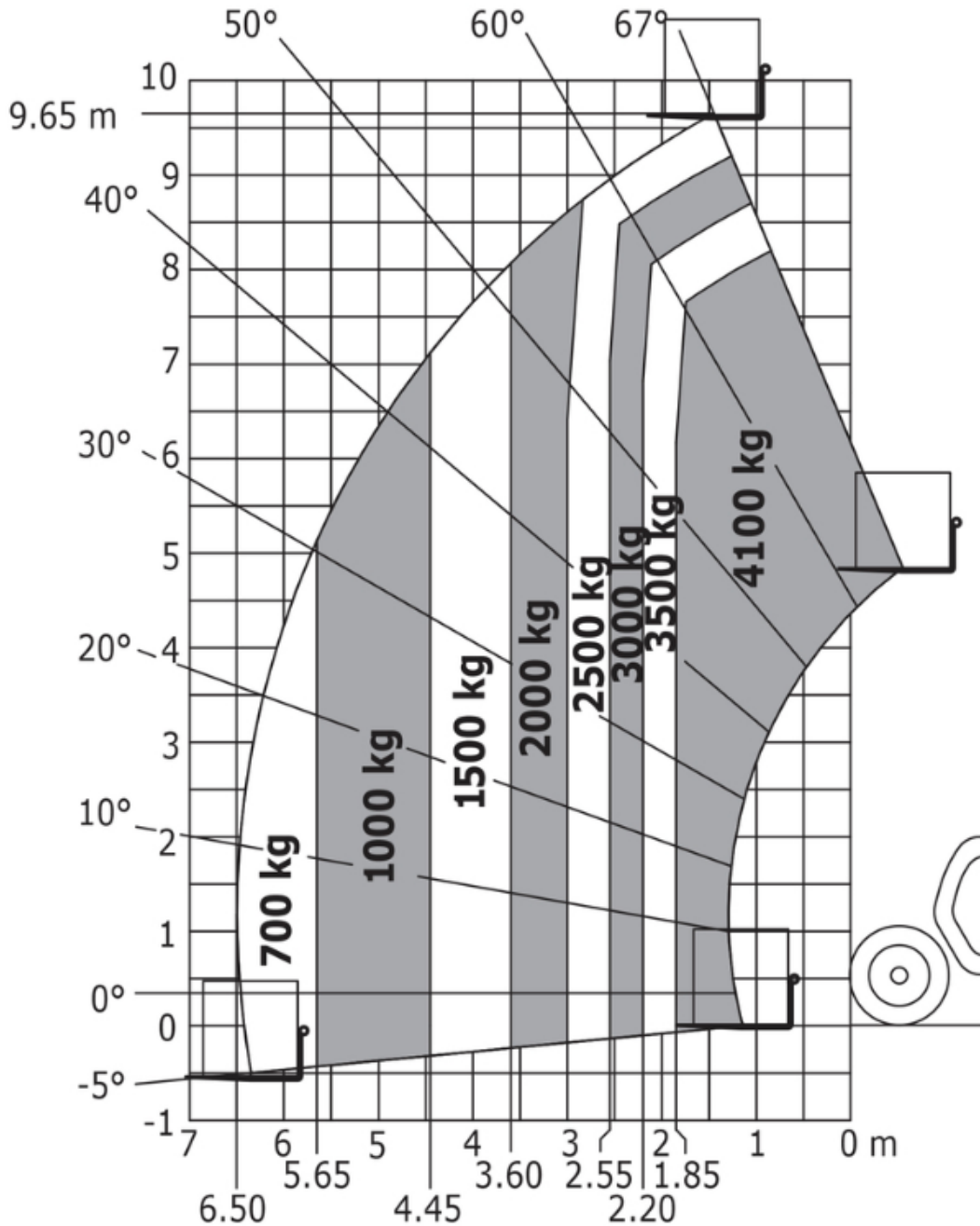
Abaque tout terrain (EN 1459 B)
