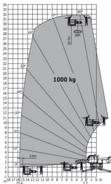
Machine sur stabilisateurs abaissés avec nacelle 1000 kg
