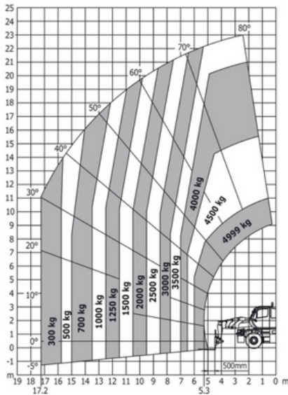
Machine sur stabilisateurs abaissés avec treuil 5000 kg
