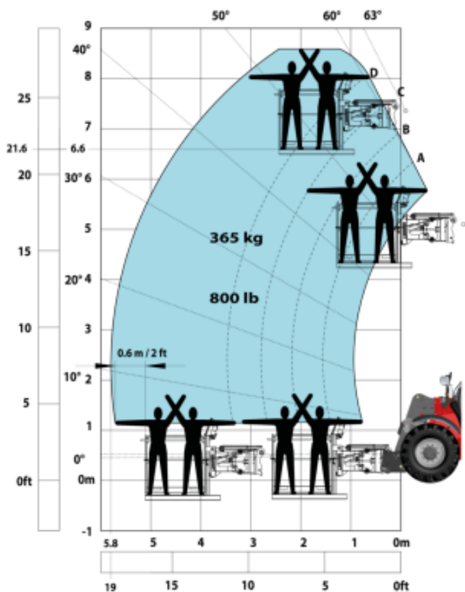
Machine sur pneus avec nacelle Métric
