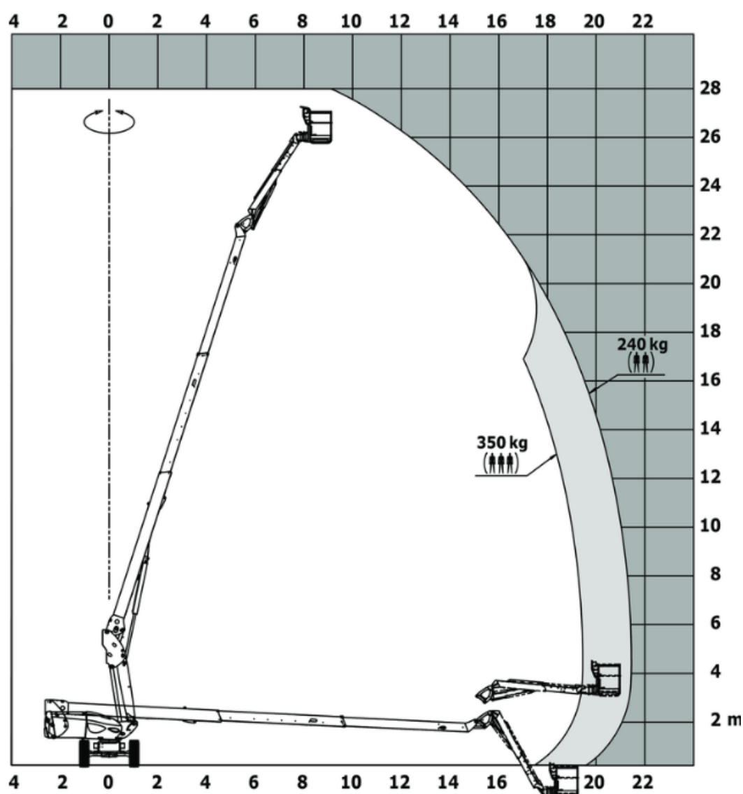
Abaque de charge pour nacelles élévatrices
