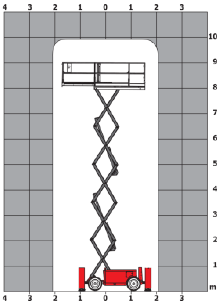
Abaque de charge pour nacelles métrique
