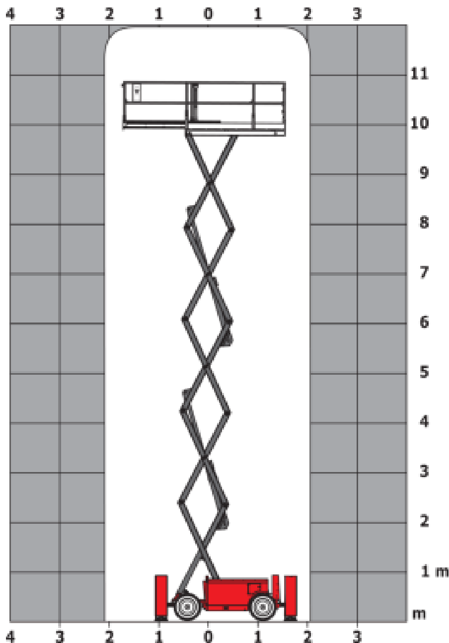
Abaque de charge pour nacelles métrique
